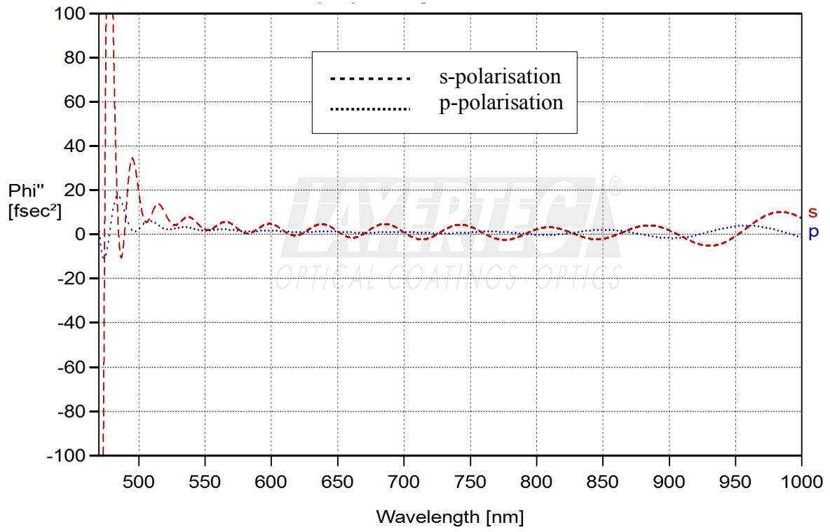
fig. 1.3: | GDD(T) < 20fsec 2 |
