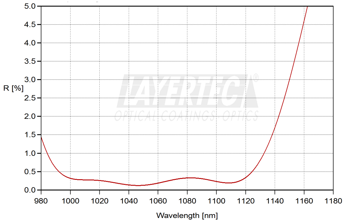
fig. 1.2: Rs (45°, 1020 - 1060nm) < 5.0%
