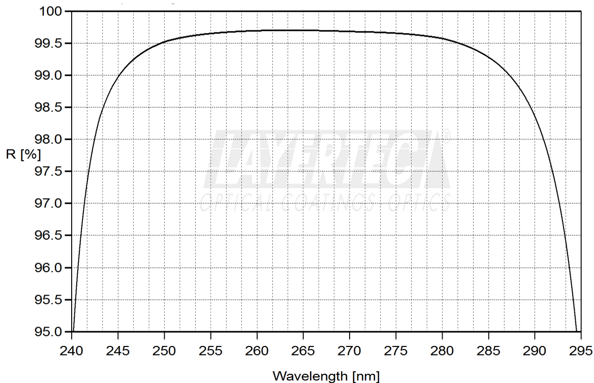
fig. 1.1: HR(0^\circ, 266\text{nm}) > 99.5\%
