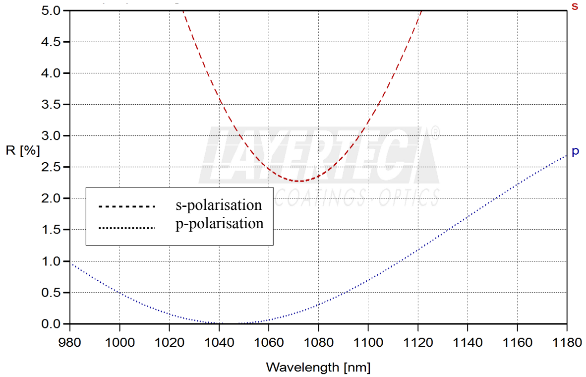
fig. 1.3: R_p(45^\circ, 1064\text{nm}) < 2.0\% + R_s(45^\circ, 1064\text{nm}) < 10.0\%
