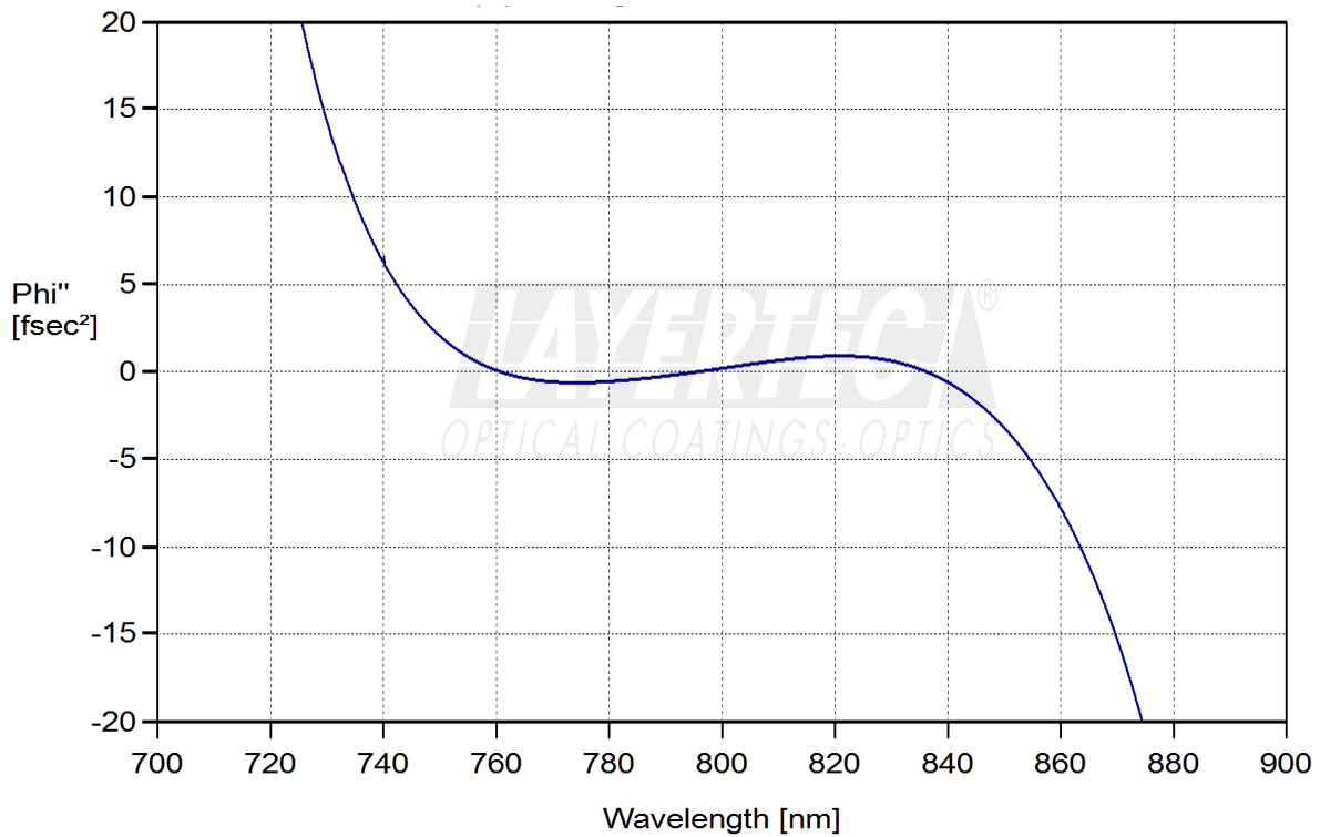
fig. 1.2: GDD < 20fsec 2
