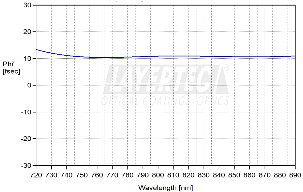
fig. 1.2: GVD < 20fsec 2
