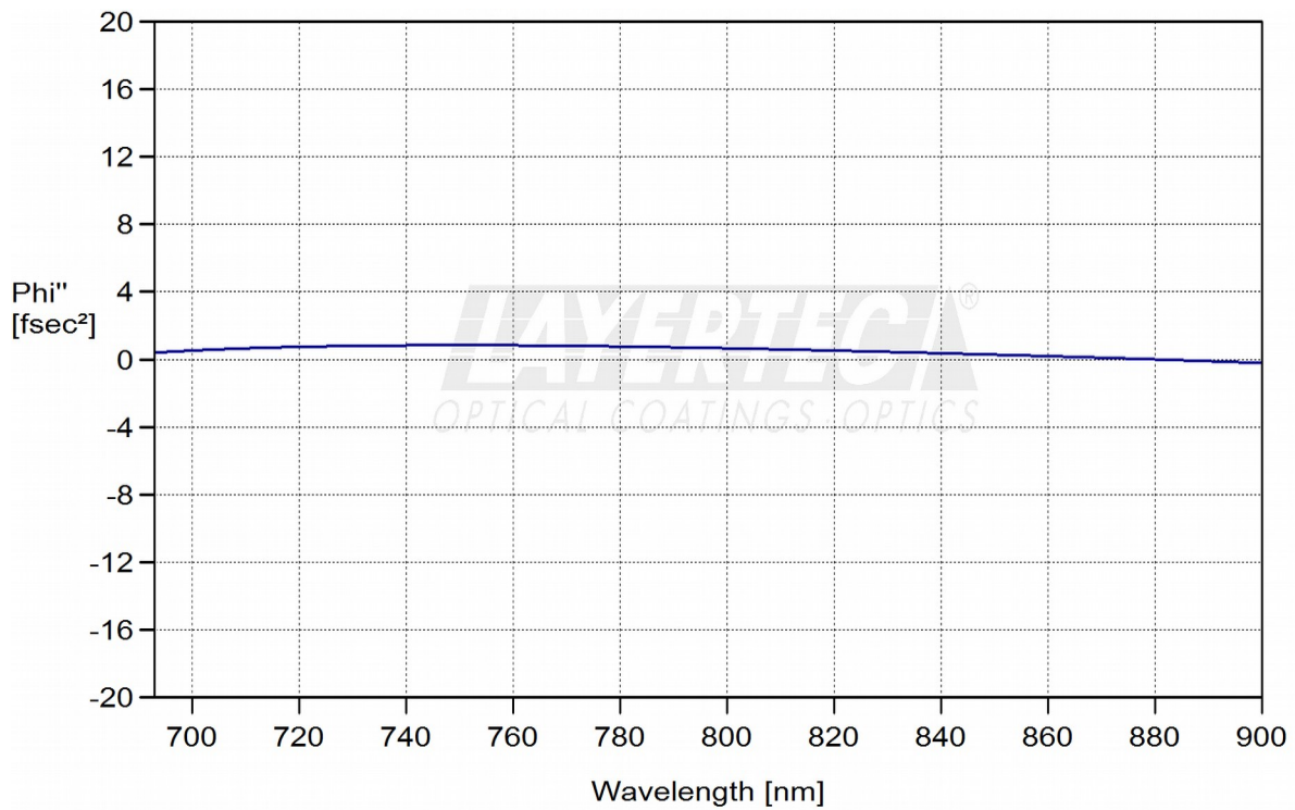
fig. 1.2: GDD < 20fsec 2
