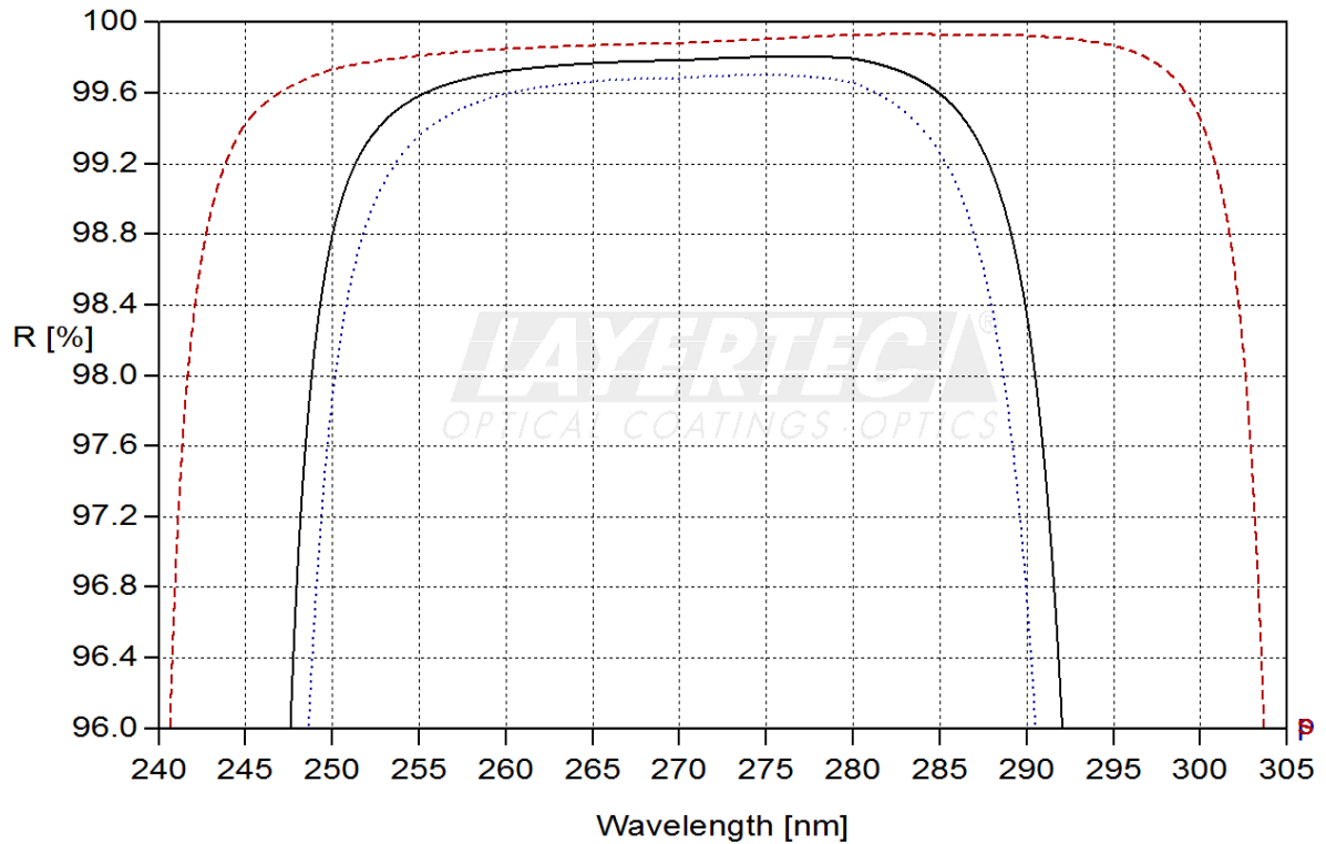
fig. 1.1: HRr(45° 270nm) >99.6%
