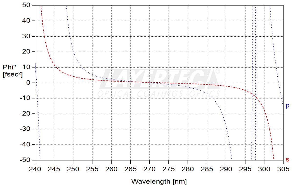
fig. 1.2: GDD-Rsp(45° 270nm) <5fs 2
