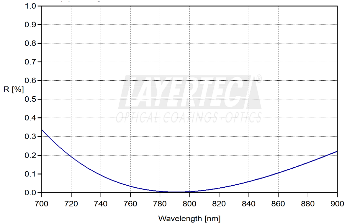
fig. 1.1: ARp (45°, 750-850nm) < 0.2%
